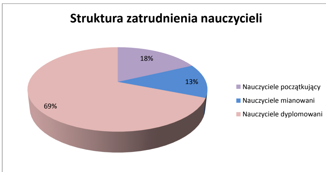
Wykres 2. Struktura zatrudnienia nauczycieli w przeliczeniu na etaty w roku szkolnym 2024/2025 – stan na dzień 30 września 2024 r.
